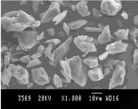
Fig. 10: SEM of Moringa oleifera gum
